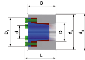
Einbauform 2
