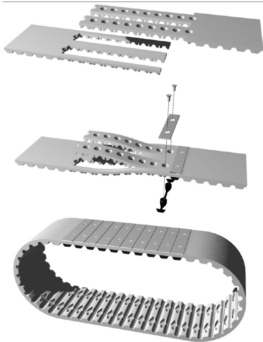
ATN-Zahnriemenschluss
