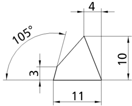
Tiefe: 98 mm Profil-Nr. 2.3.3.011.010
