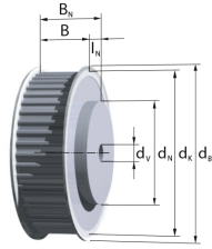
Standardausführung 6F
