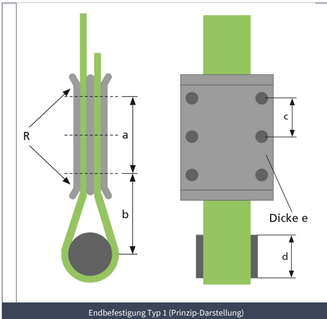
Endbefestigung Typ 1 (Prinzip-Darstellung)
