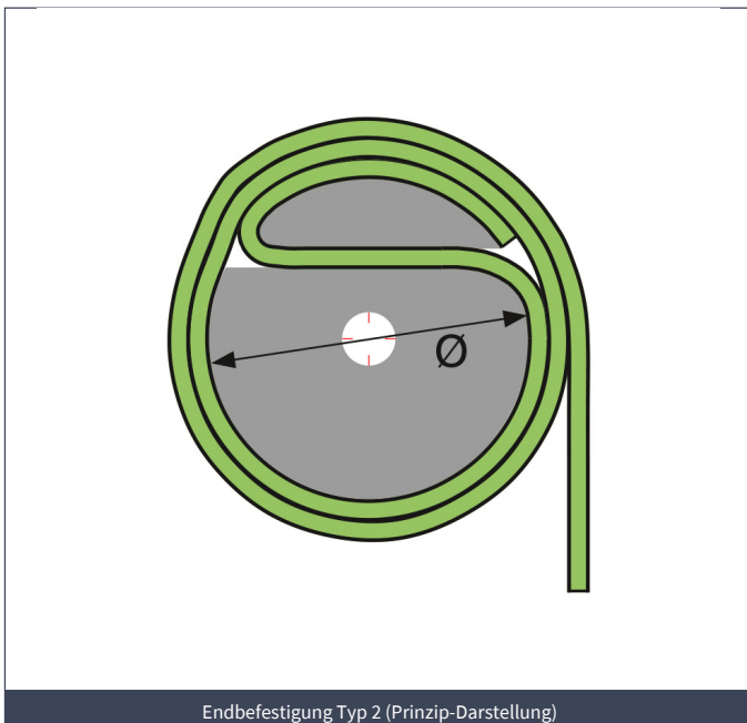
Endbefestigung Typ 2 (Prinzip-Darstellung)
