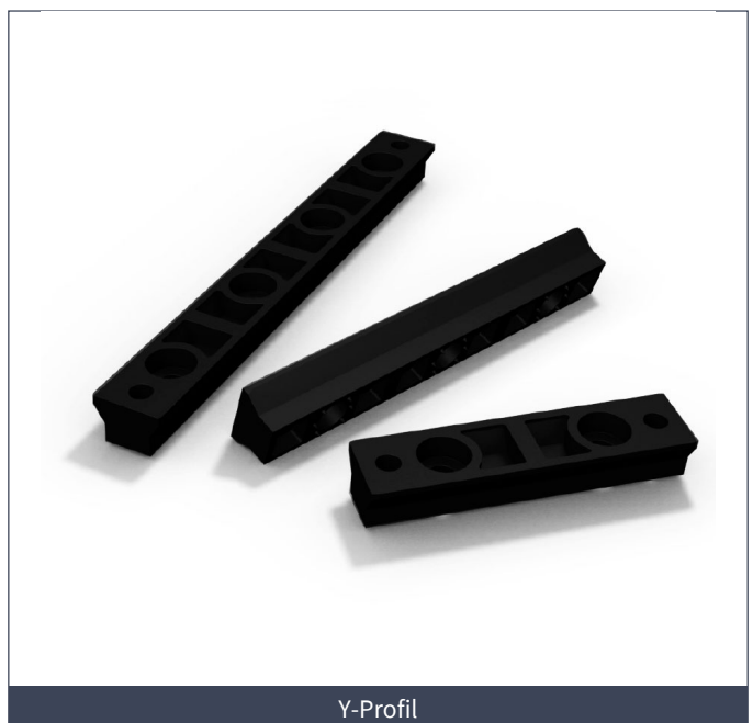
Breite 75 mm, Profil-Nr.: 1.001.009
