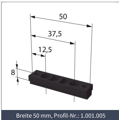
T-Profil
