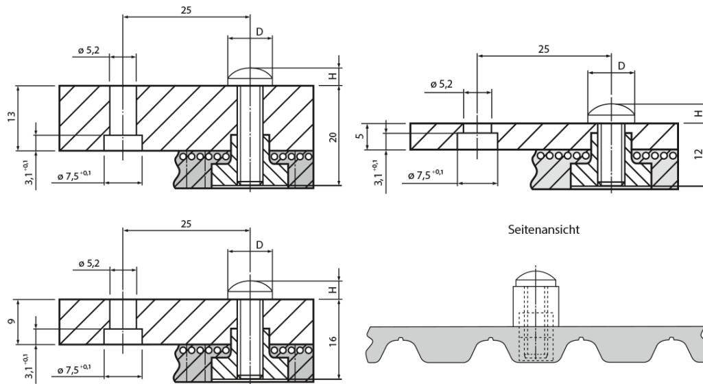
Anschlussgeometrie ATN 20 (Schnitt durch Riemenzahn)
