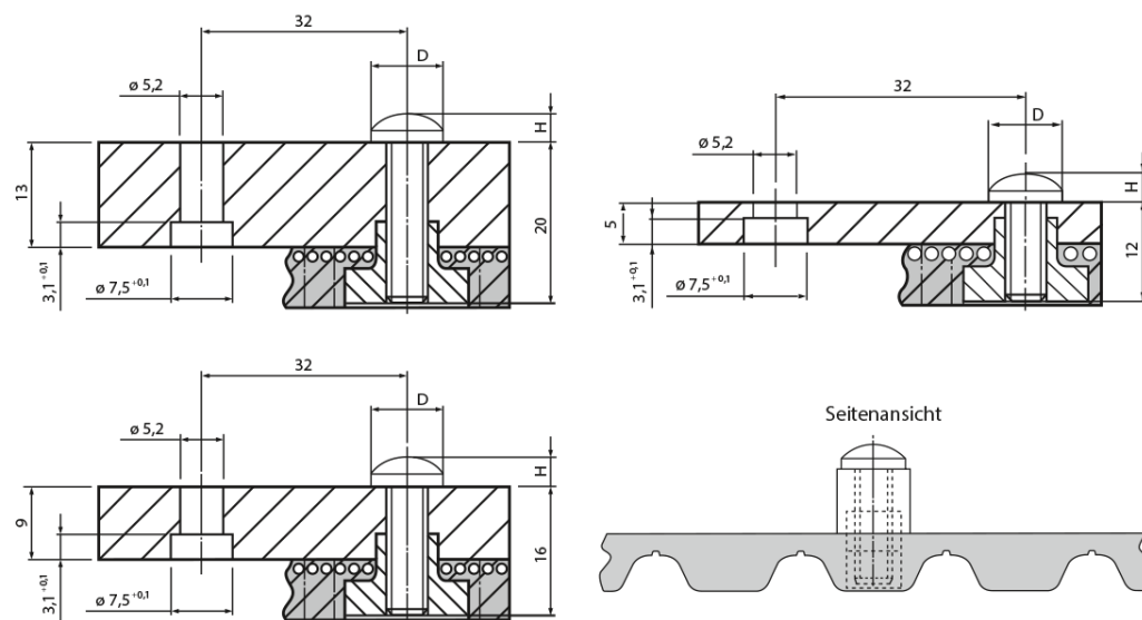
Anschlussgeometrie ATNS 20 (Schnitt durch Riemenzahn)
