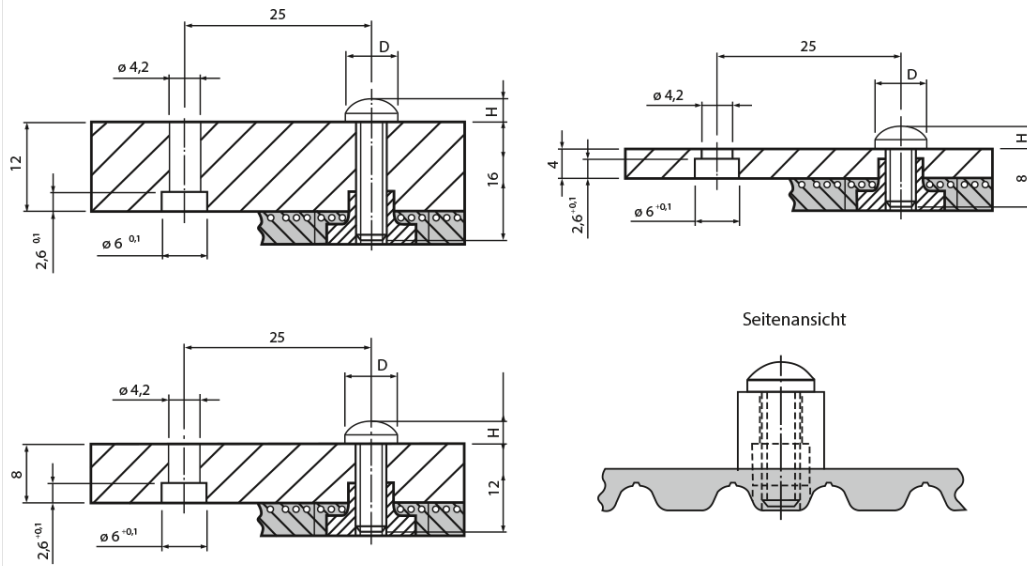
Anschlussgeometrie ATN10 / ATN10K6 / ATN 12,7 / ATN12,7K6 (Schnitt durch Riemenzahn)
