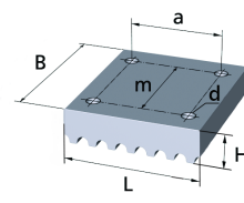
Klemmverbinder für einseitige Riemeneinspannung
