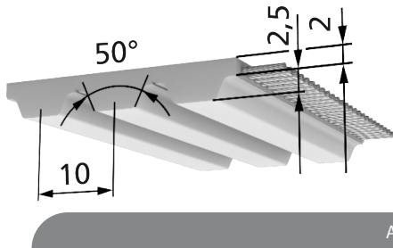
Verstärkter Riemenrücken
