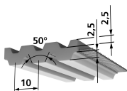
Doppelt verzahnt
