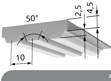
Ausführung T
